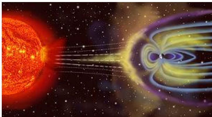
شکل ۲-۱) مگنتوسفر
