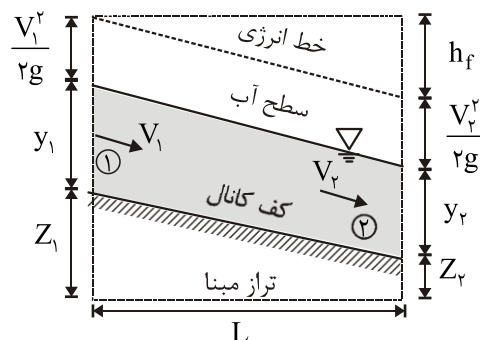
شکل ۱-۱: «مشخصات یک مقطع از یک کانال باز»
