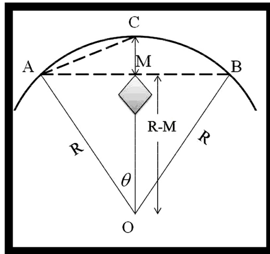
(شکل ۷-۲) وجود مانع در قوس افقی
